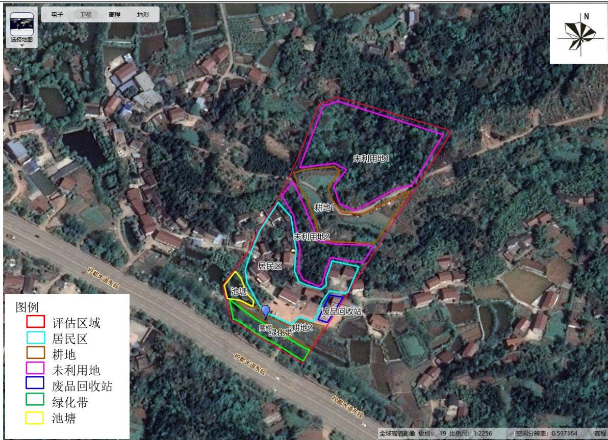
图 3.5-1 地块内平面布局图
