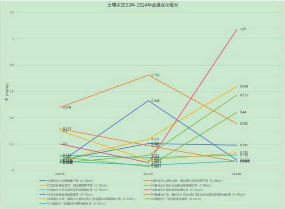
图8.3-2 土壤汞2022年-2024年含量变化表
