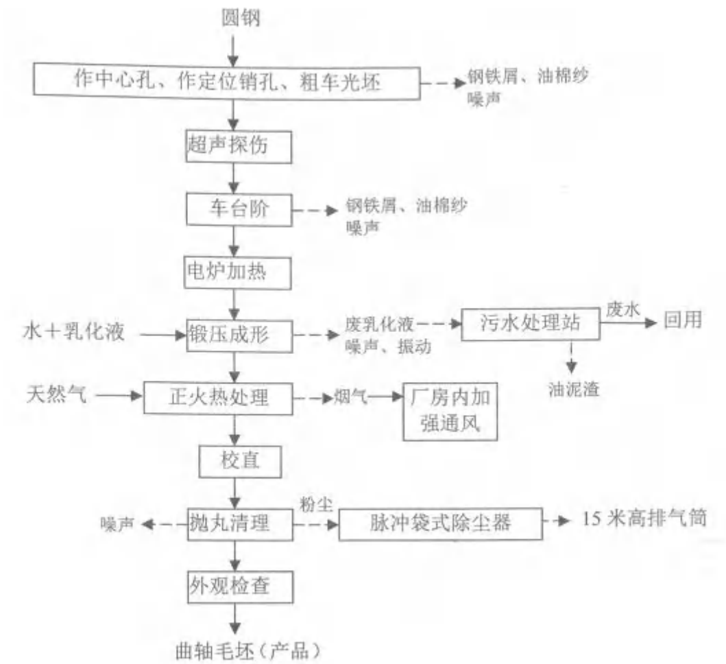
图 4.2-1 曲轴锻造毛坯生产工艺及产污环节图
