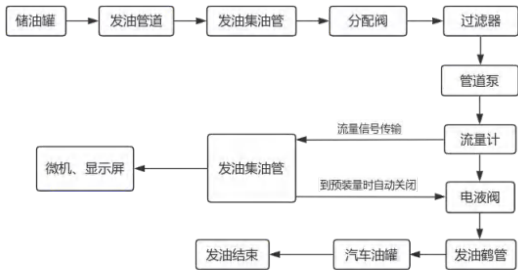
6.2.2-2 发油工艺图
